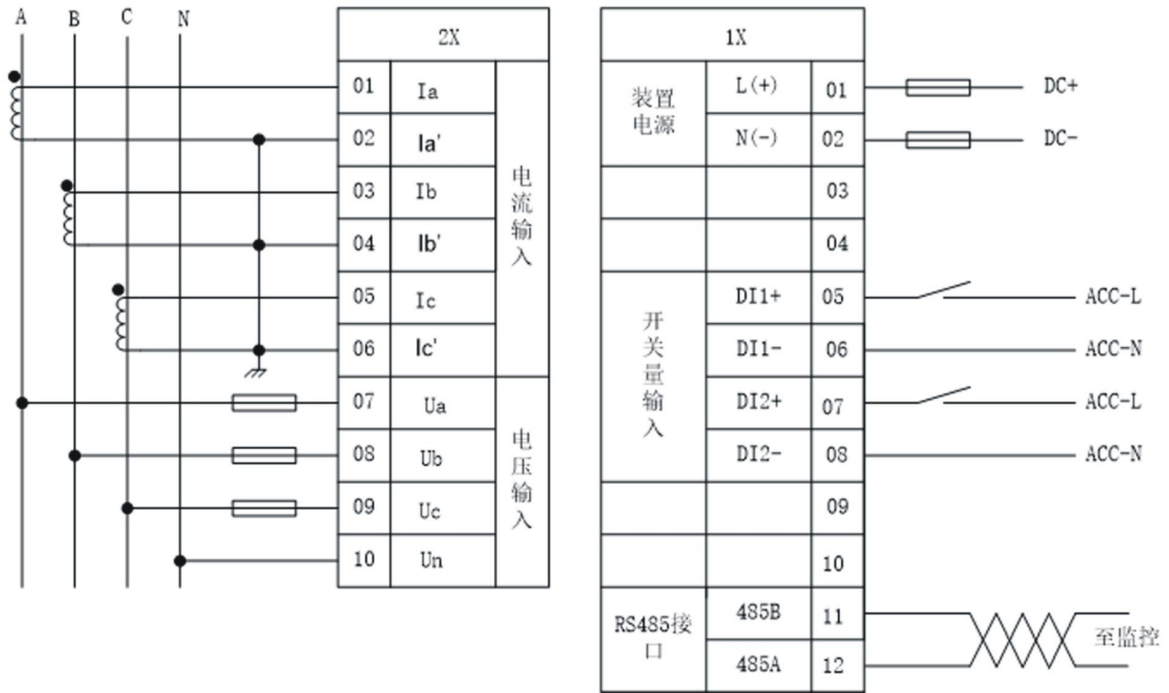
YW-331A电力多功能仪表
