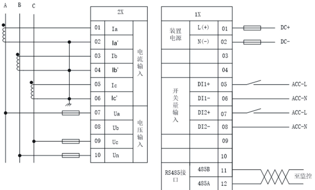
YW-331A电力多功能仪表
